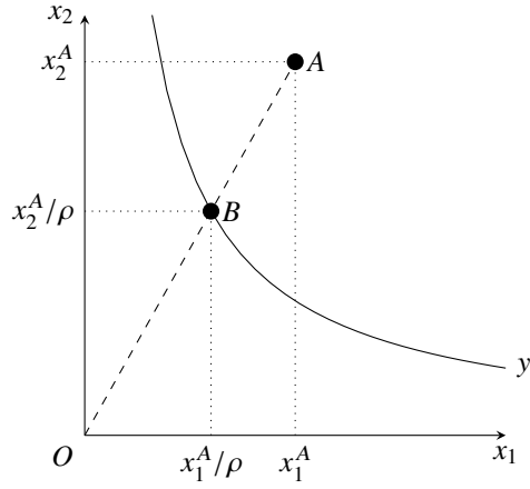
図1 等量曲線と距離関数
